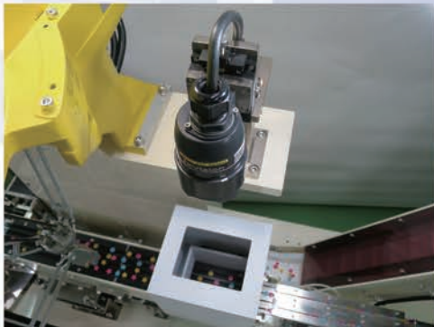
2種類の形状の部品を1台の パーツフィーダで選別、振分、整列
