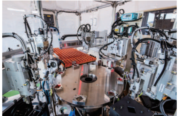
組立機
